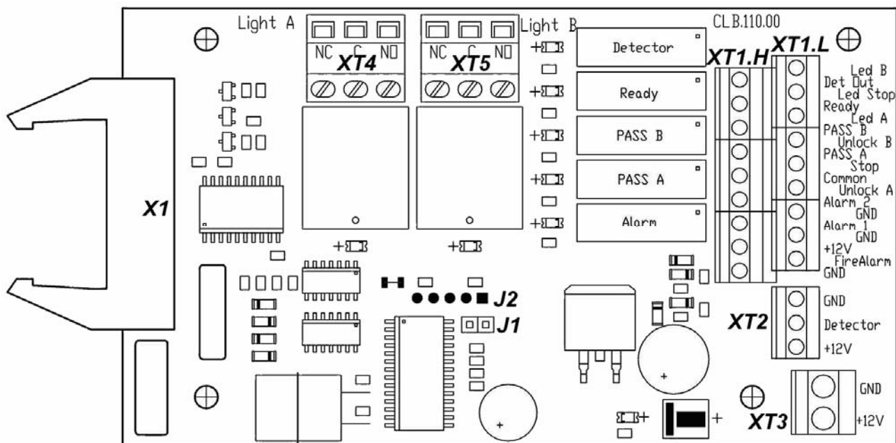
Рисунок 2. Внешний вид платы
