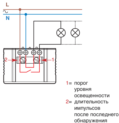
Тип 18.21 / 18.31 / 18.31...0031
