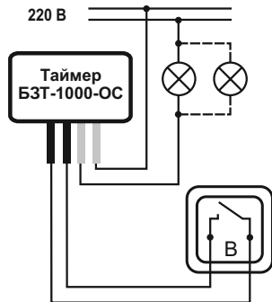
Рис.1. Схема монтажа
