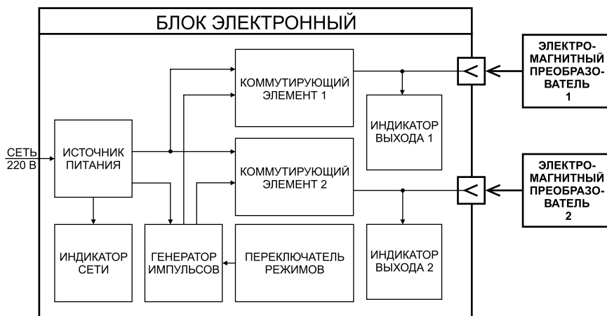
Рис. 1 Структурная схема импульсатора ЭИ-102
